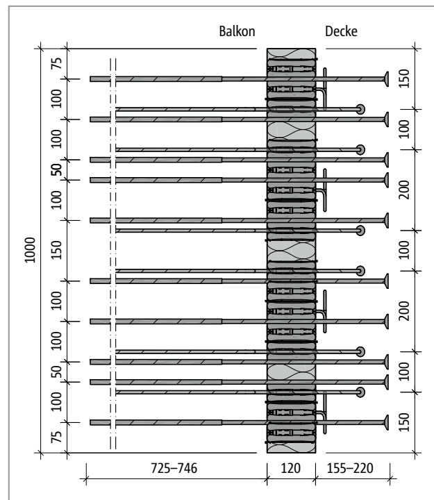
Abb. 122: Schöck Isokorb® XT Typ K-U-M4: Produktgrundriss
