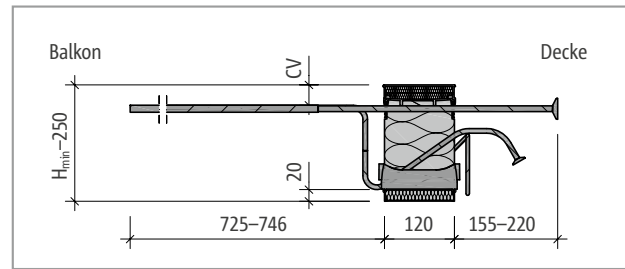
Abb. 120: Schöck Isokorb® XT Typ K-U-M4: Produktschnitt
