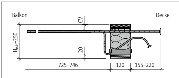
Abb. 119: Schöck Isokorb® XT Typ K-U-M2: Produktschnitt
