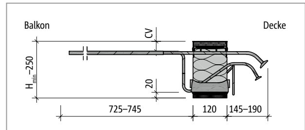
Abb. 124: Schöck Isokorb® XT Typ K-O-M4: Produktschnitt
