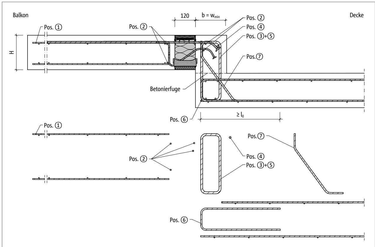
Abb. 132: Schöck Isokorb® XT Typ K-O: Bauseitige Bewehrung für Balkon mit Höhenversatz nach oben mit minimaler Bauteilabmessung ( w_{\text{vorth}} = w_{\text{min}} )
