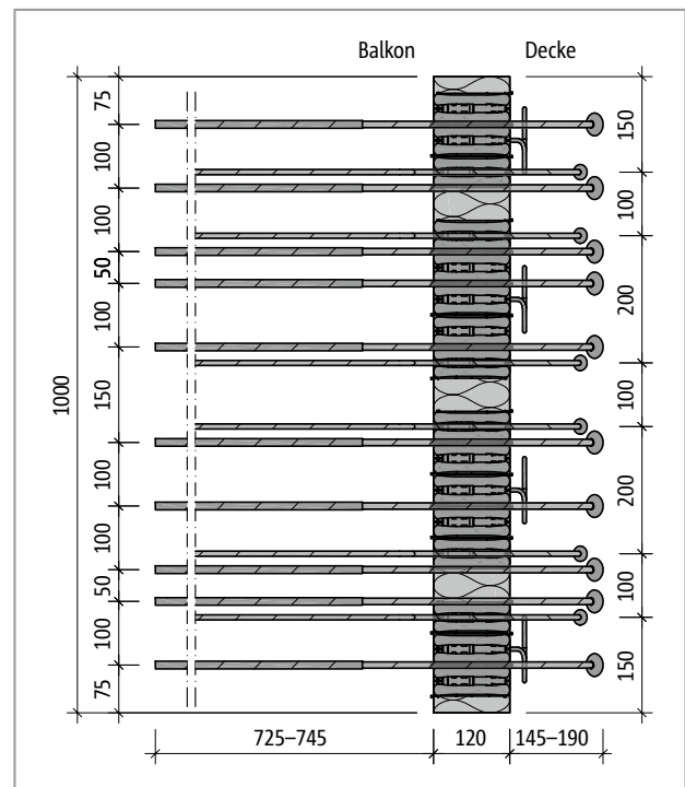
Abb. 126: Schöck Isokorb® XT Typ K-O-M4: Produktgrundriss
