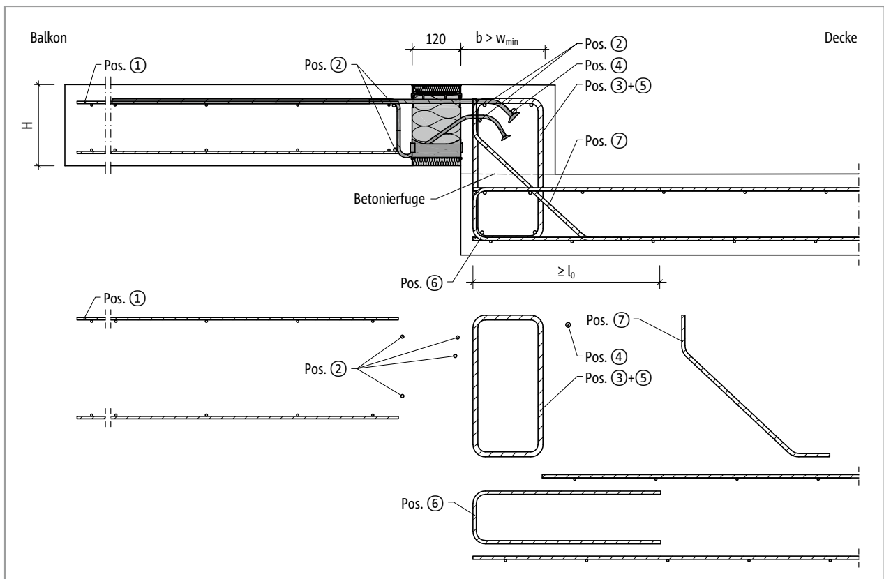
Abb. 133: Schöck Isokorb® XT Typ K-O-F: Bauseitige Bewehrung für Balkon mit Höhenversatz nach oben mit größerer Bauteilabmessung ( w_{\text{vorth}} > w_{\text{min}} )
