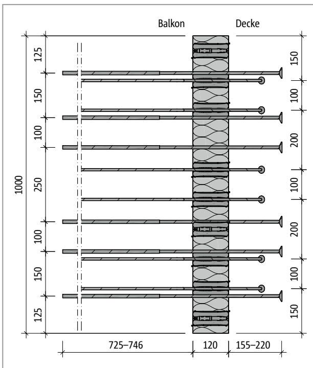
Abb. 121: Schöck Isokorb® XT Typ K-U-M2: Produktgrundriss
